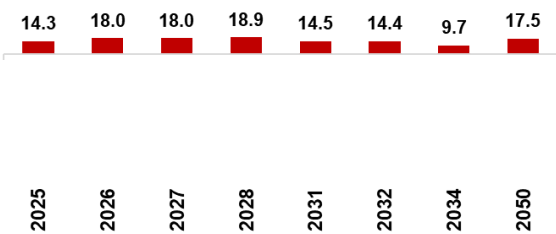
Gráfica 4: Variación diaria TES Tasa Fija (pbs)
